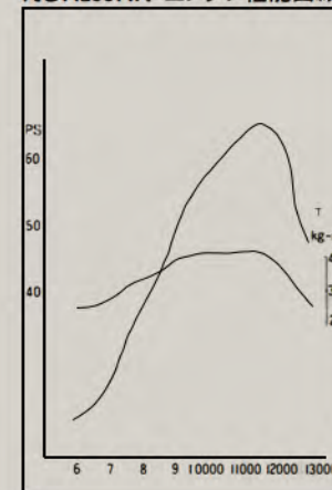
NSR250RK エンジン性能曲線
