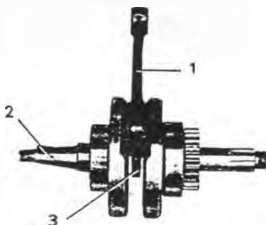
Afbeelding 33. 1. Naaldlager 2. Naaldlagerkooi 3. Lepel
