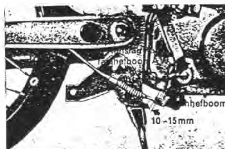
Vrije speling tussen remhefboom en aanslag.
