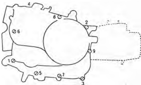
Afbeelding 9. Volgorde voor het aandraaien van de kruiskopschroeven
