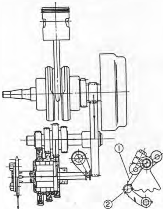
Afbeelding 41. Stand 3e versnelling
