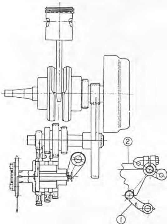
Afbeelding 39. Stand 1e versnelling
