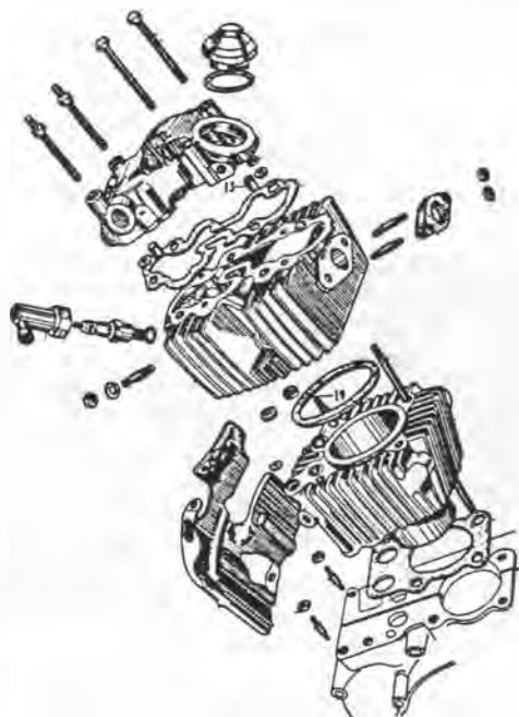
Afbeelding 4. Cylinder en Cilinderkop
