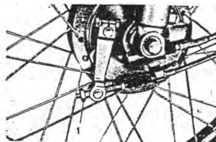
Stelmoer (C) van de voorrem. 1. — Stelmoer.
