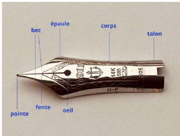
Détails d'une plume 14 carats (Sailor)
