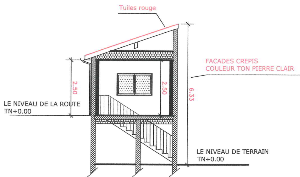
COUPE AA - 1/100
