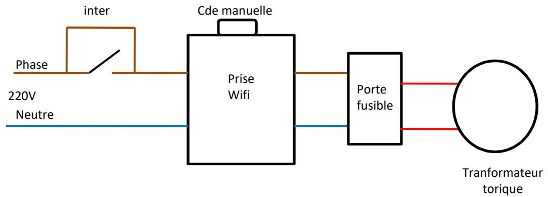
Schéma modifié
