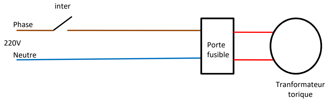
Schéma actuel
