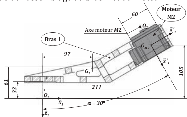
Figure 15 : Dessin de l'assemblage du bras 1 et du moteur M2
