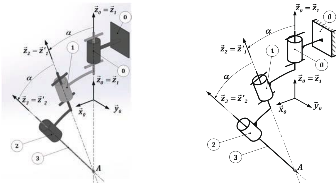
Figure 7 : Modèle cinématique de la solution architecturale proposée par l'équipe RobioSS de l'institut de recherche Pprime. Les schémas sont proposés pour une configuration particulière :
