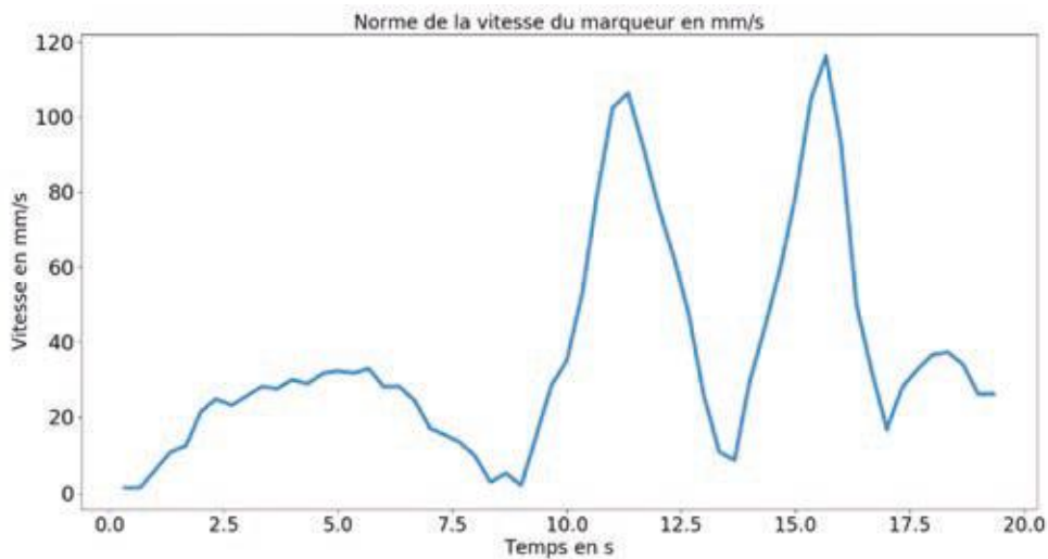
Figure 5 : Norme (en \text{mm} \cdot \text{s}^{-1} ) de la vitesse de l'effecteur au cours du temps
