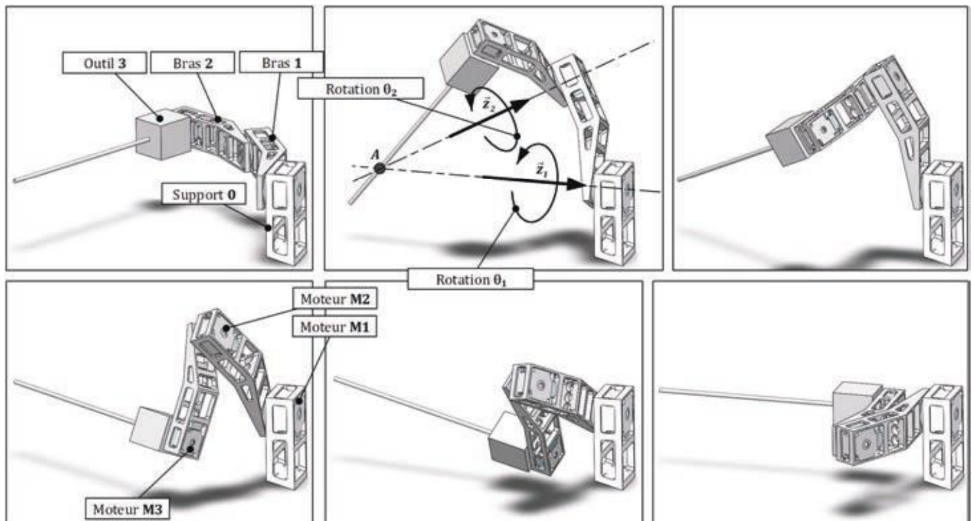
Figure 17 : Description du mouvement critique du robot
