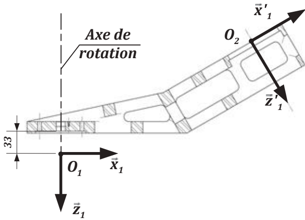
Figure 12 : Extrait du dessin de définition du bras 1
