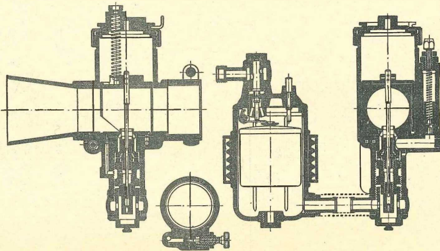
Sezione schematica
