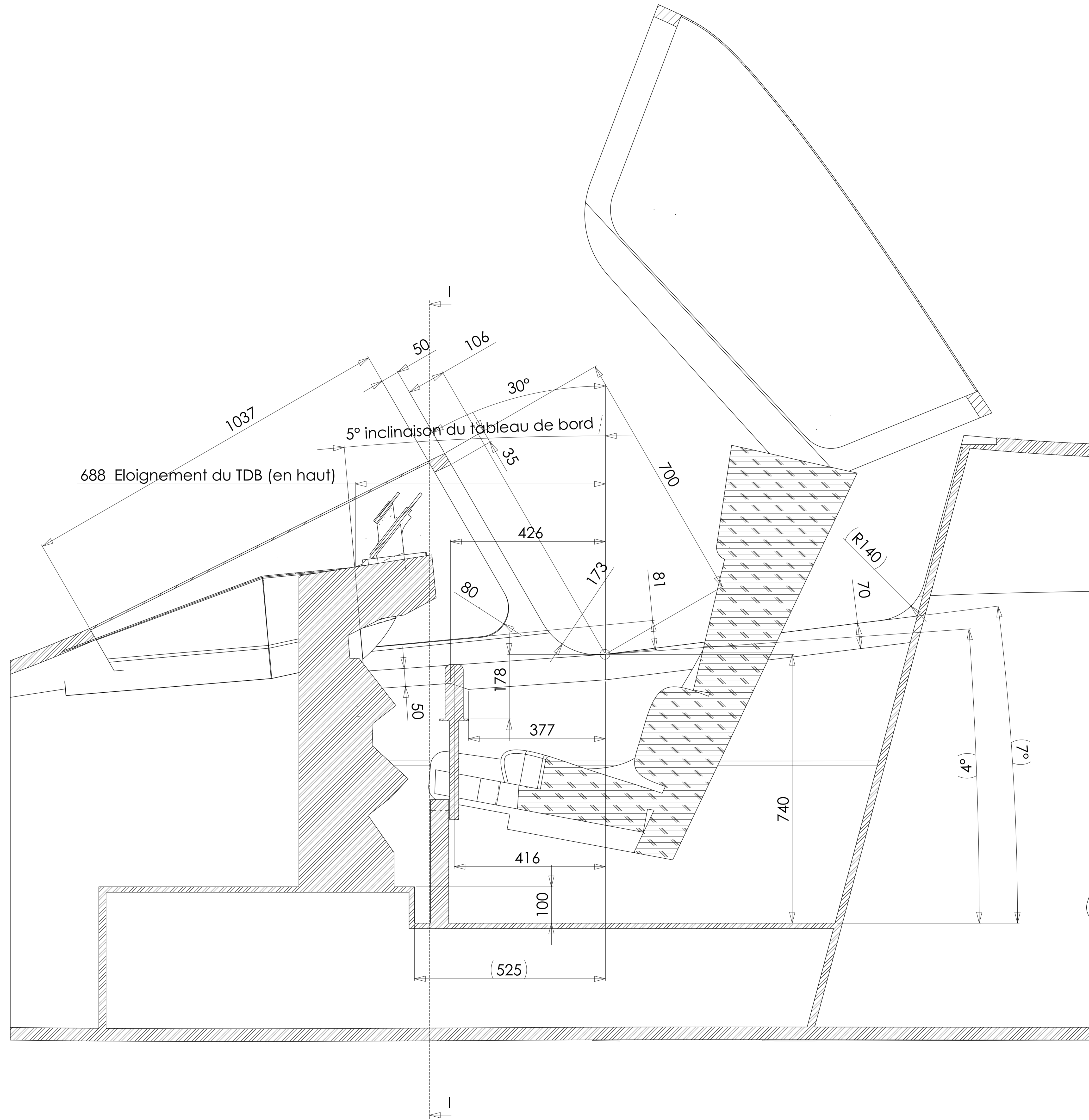
COUPE B-B ECHELLE 1 : 5
