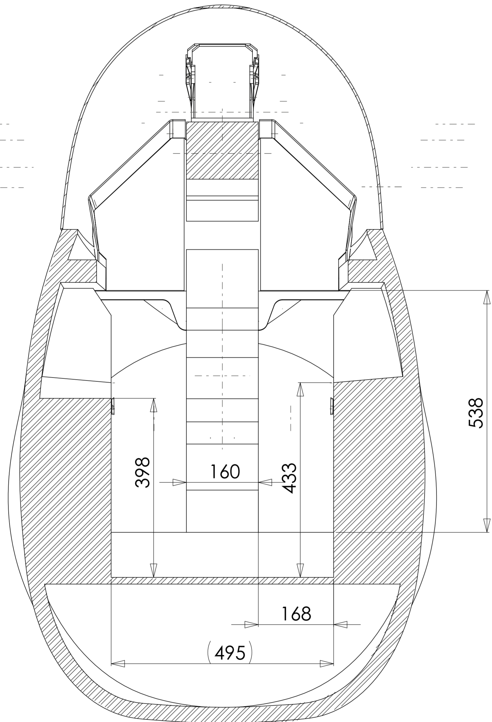
COUPE I-I ECHELLE 1 : 5
