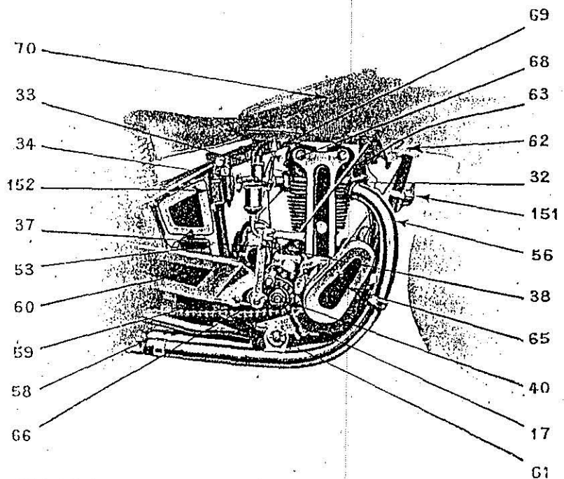
BLOC-MOTEUR A CULBUTEURS MONTÉ DANS LE CADRE VU DU COTÉ DROIT
