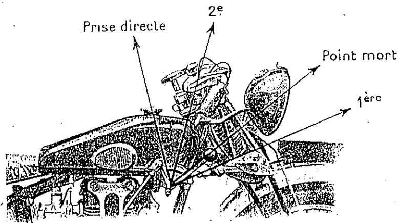
POSITION DU LEVIER A MAIN DES VITESSES
