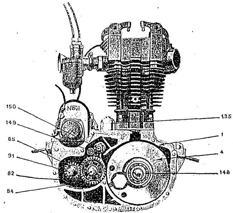
BLOC-MOTEUR A CULBUTEURS VU DU COTÉ DROIT (Le couvercle enlevé)
