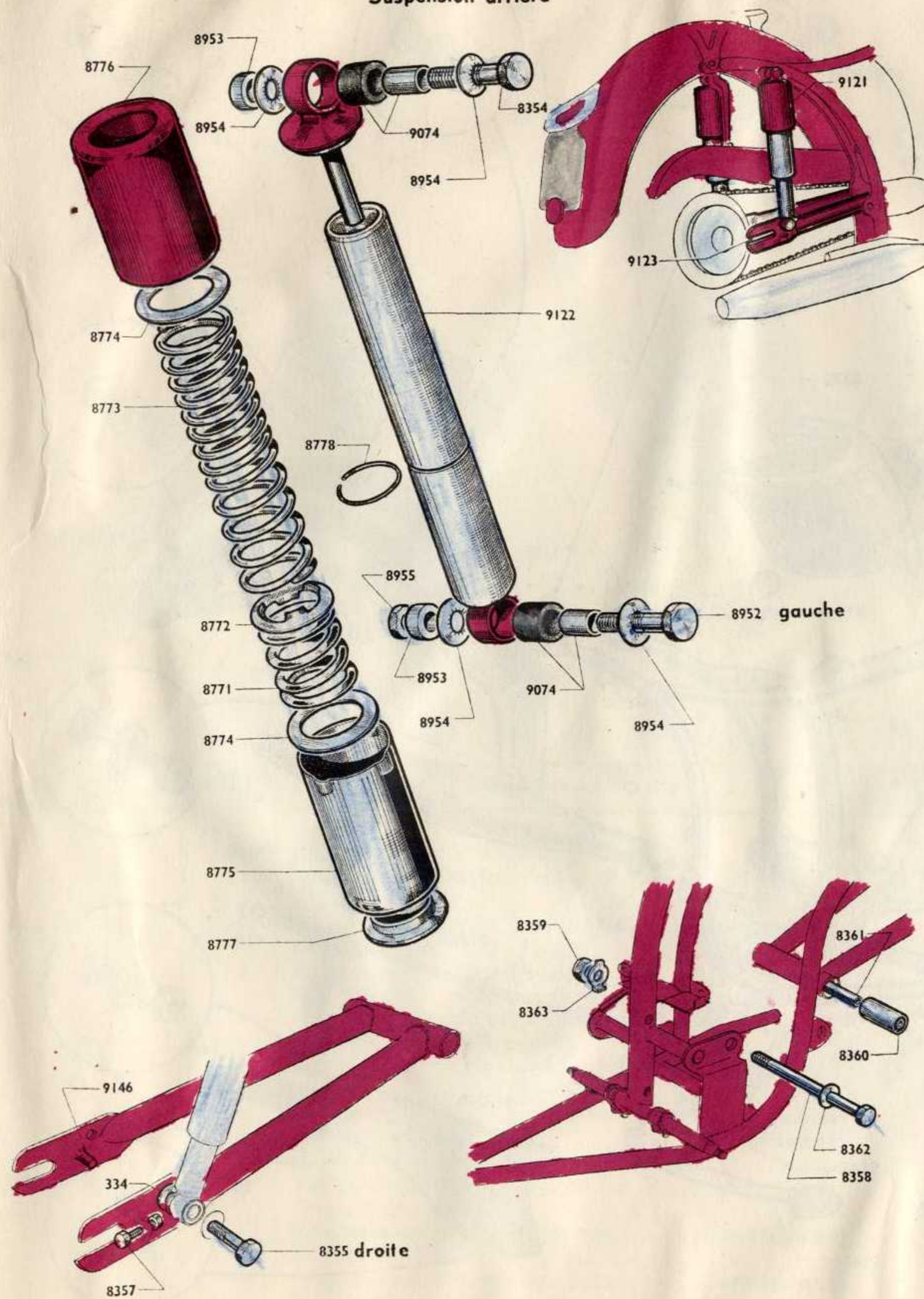
Suspension arrière
