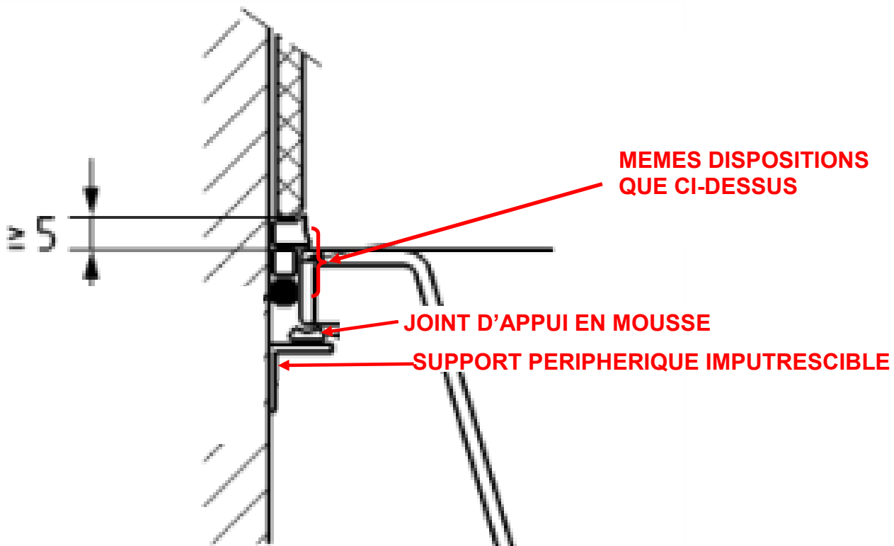
CAS D'UN BAC A DOUCHE OU BAIGNOIRE ACRYLIQUE
