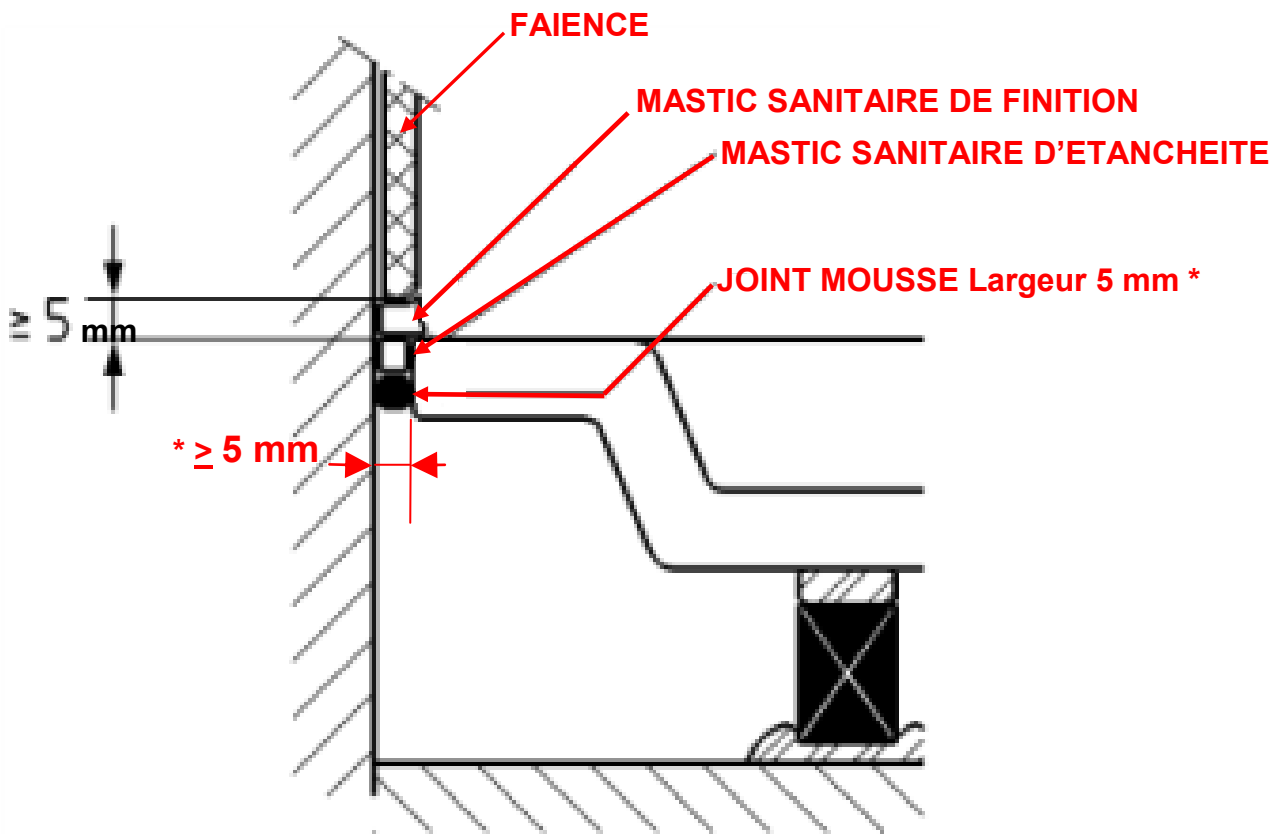
CAS D'UN BAC A DOUCHE CERAMIQUE OU BAIGNOIRE ACIER, FONTE
