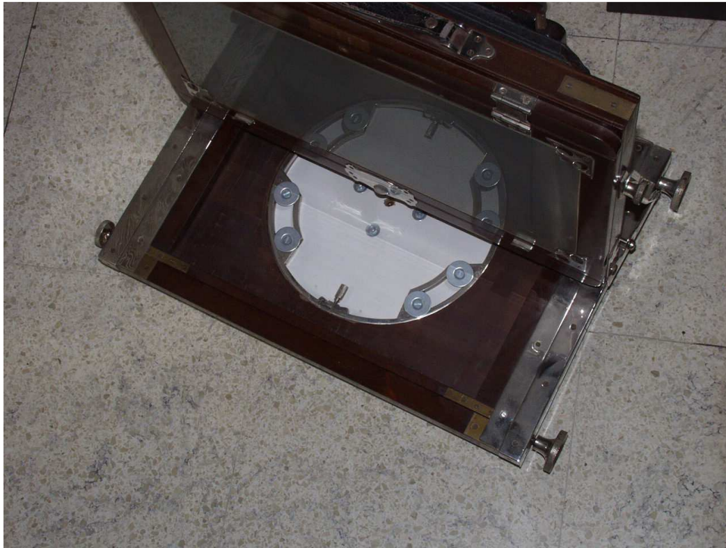
Fixation du nouveau support – vue de dessus – rondelles « couvreur »
