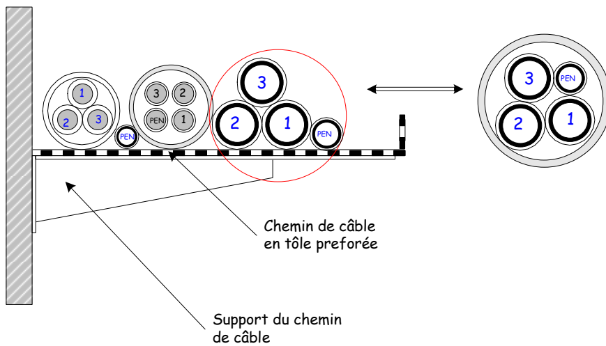
Exemple de canalisation électrique
