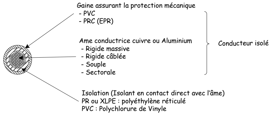
Coupe d'un câble monoconducteur unipolaire
