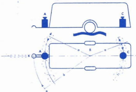
Fig. n° 10 - Charge incorrecte : les masses étant situées aux extrémités de la caravane entraînent une tendance aux lacets.
